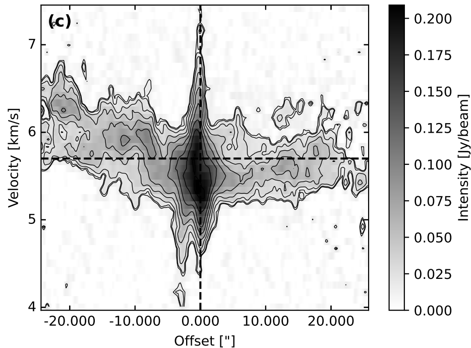
\text{H}_2\text{CO} (3 0,3 -2 0,2 ) PV Diagram
